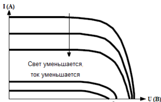
Свет уменьшается, и напряжение холостого хода уменьшается
