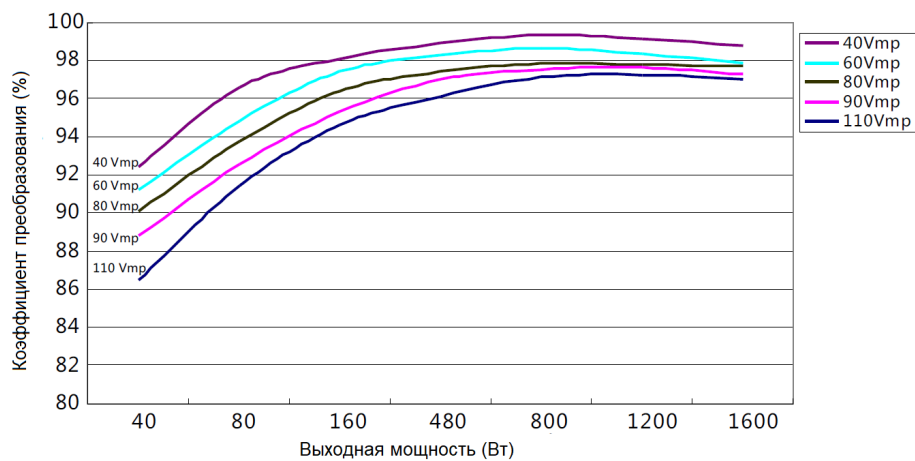
MPPT 24В Эффективность преобразования (24В батарея)
