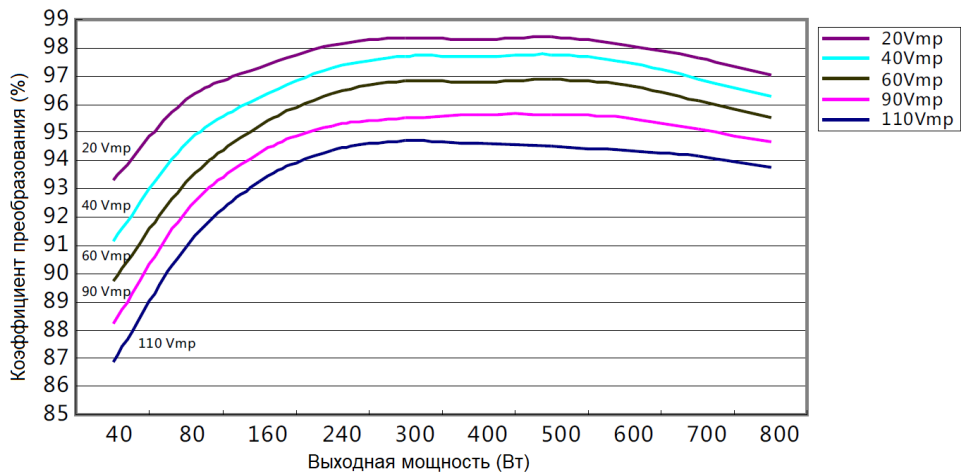
MPPT 12 В Эффективность преобразования (12В батарея)
