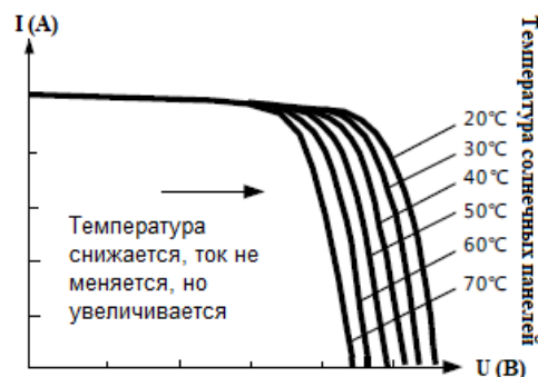
Повышается температура, уменьшается напряжение холостого хода
