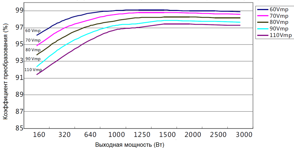
MPPT 48В Эффективность преобразования (48В батарея)
